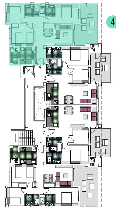
(PLANTA 4º)
