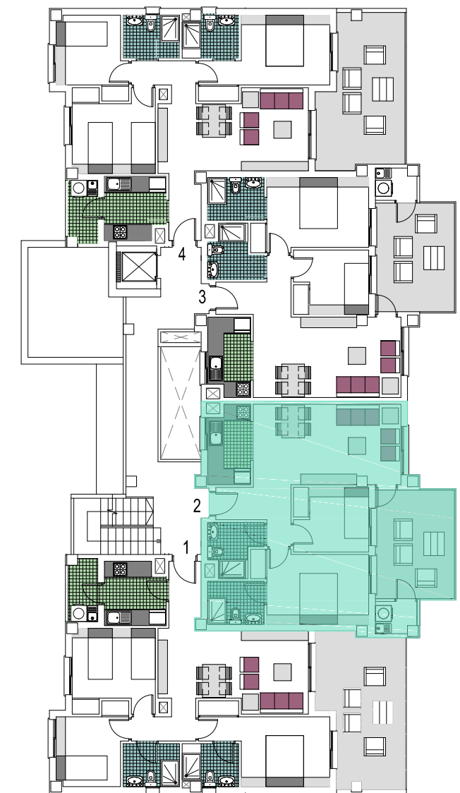
(PLANTA 1º)
