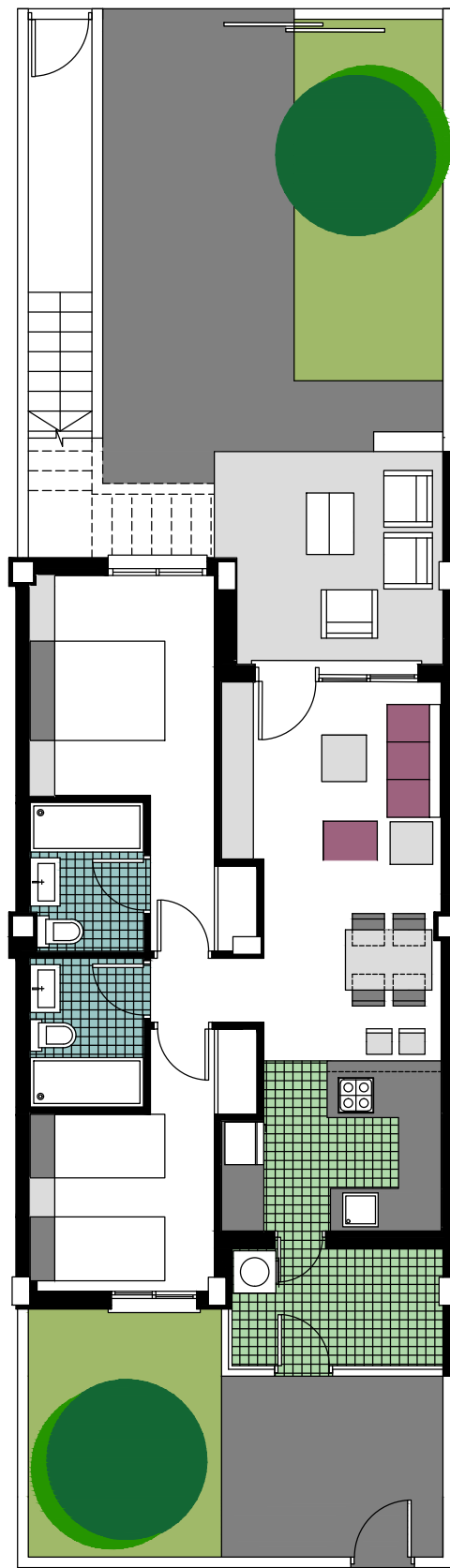
PLANTA BAJA
